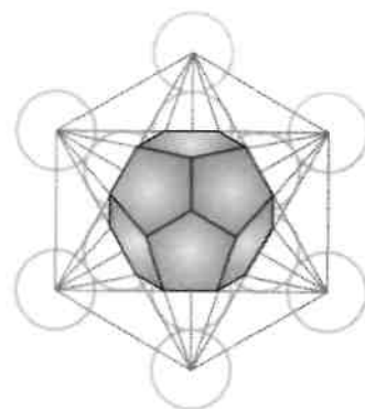
Illustration 6-21a. Dodécaèdre rendu plus solide.
