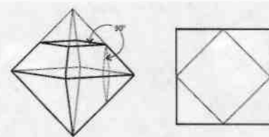
Illustration 6-40. Observation de la facette (à droite) créée en retranchant les six pointes d'un octaèdre. À gauche, nous présentons ce dernier avec une seule pointe tronquée, ainsi qu'une autre en pointillé à 90 degrés de la première.
