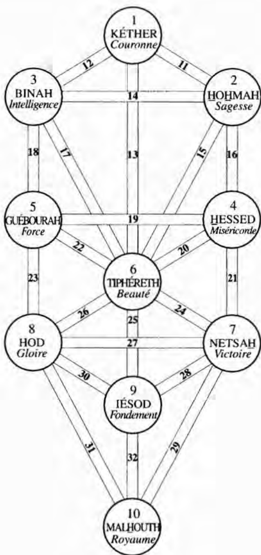
Arbre séphirotique
